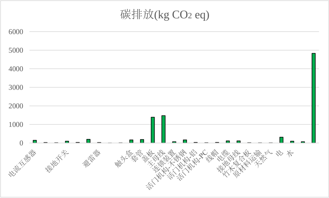
图 6 生命周期各物质的碳足迹的分析结果
